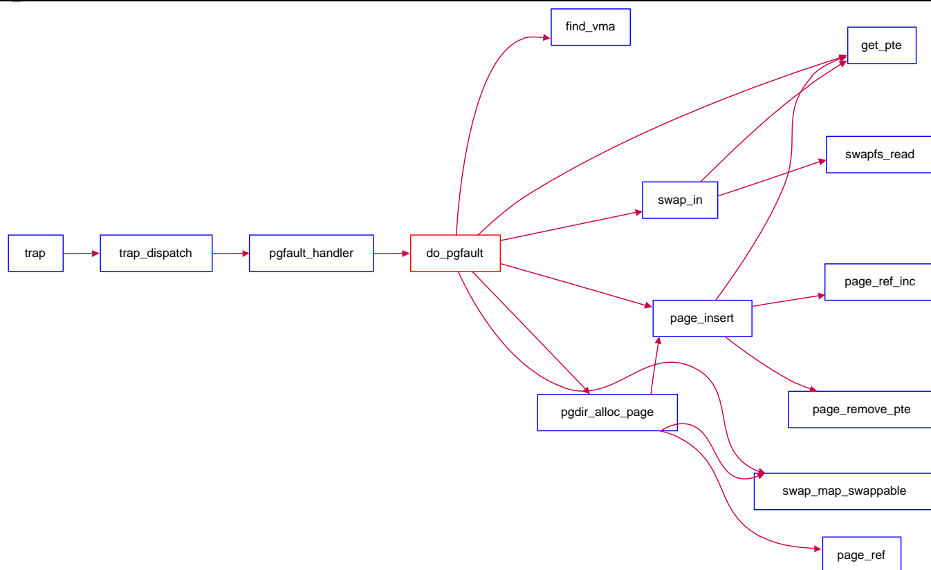
图 do_pgfault的调用关系图
